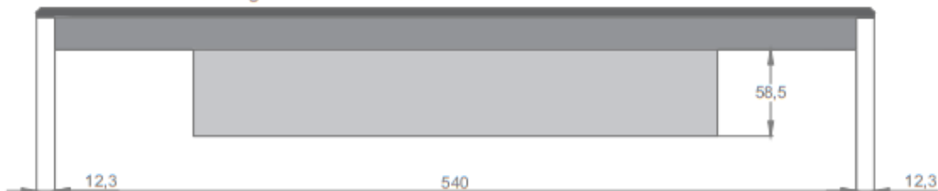
Dima di Foratura Consigliata 542mm x 333mm
